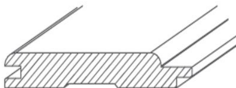
Профил Softline
